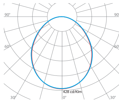
Krzywa rozsytu światłości wybranej oprawy LIGHT STEP NT / sD cd/klm — C0 - C180 — C90 - C270
