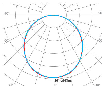
Krzywa rozsyłu światłości wybranej oprawy QUATTRO SLIM K / D cd/klm — C0 - C180 — C90 - C270
